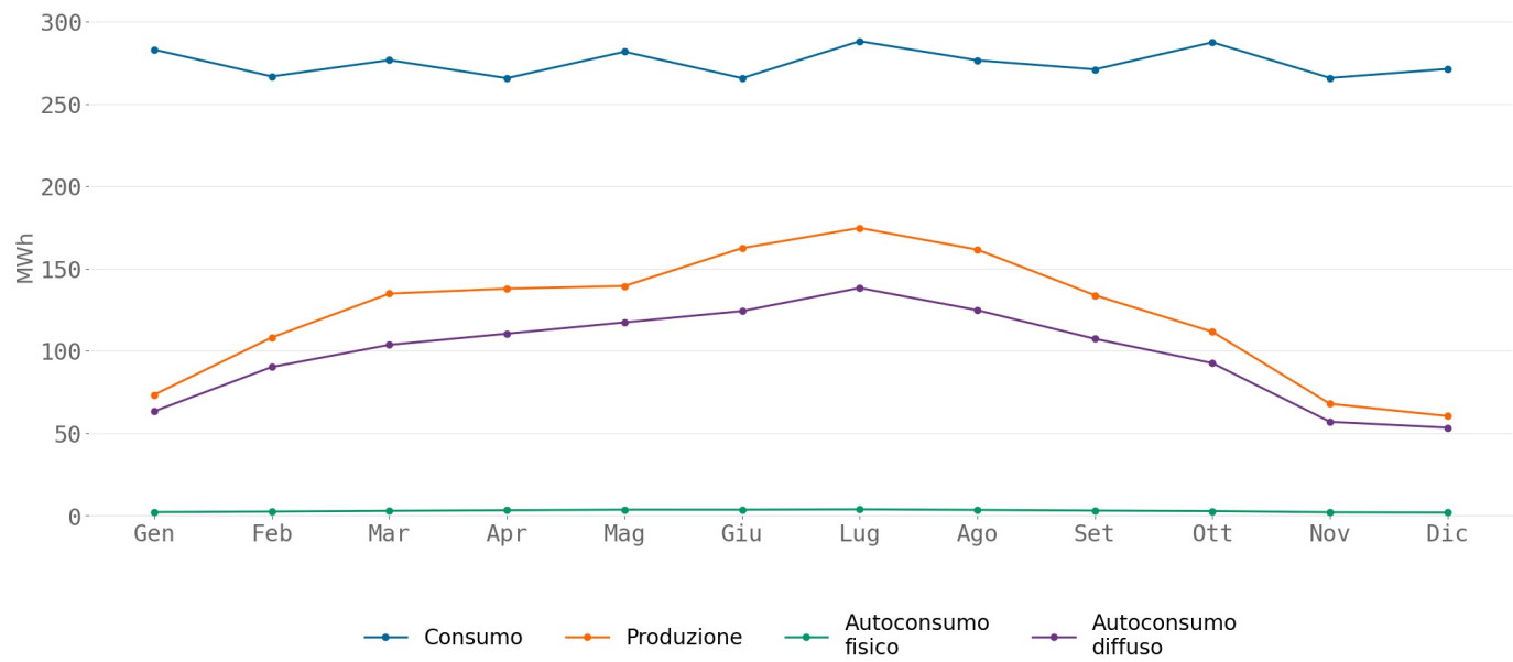
Performance energetiche mensili della configurazione - anno 2028
