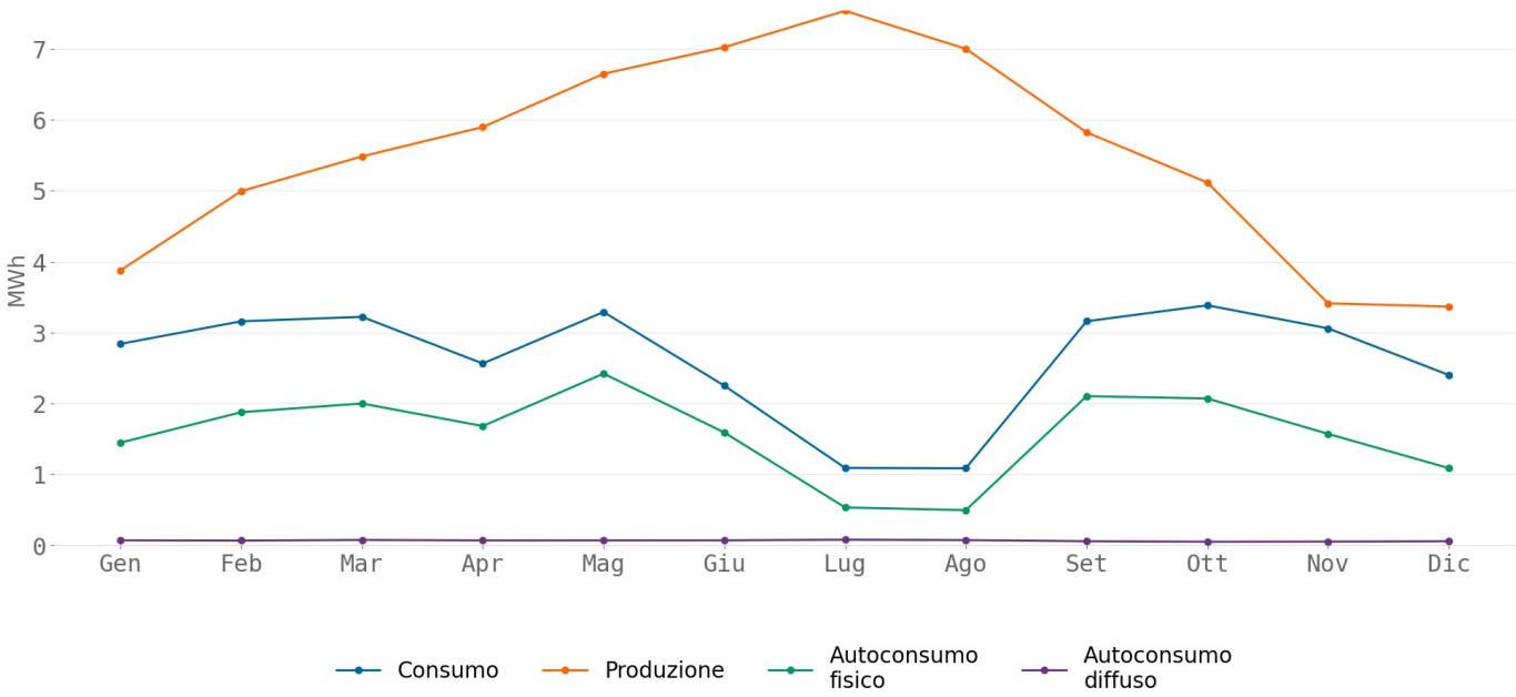
Performance energetiche mensili della configurazione - anno 2028
