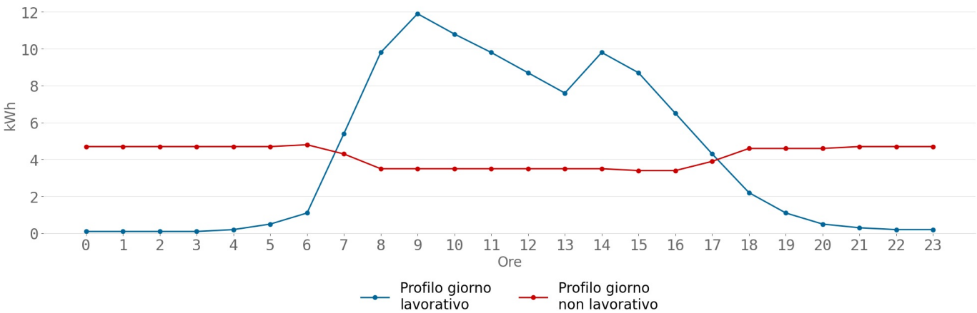
Profilo di consumo orario: CER_Fluminimaggiore (Officina_Comunale)
