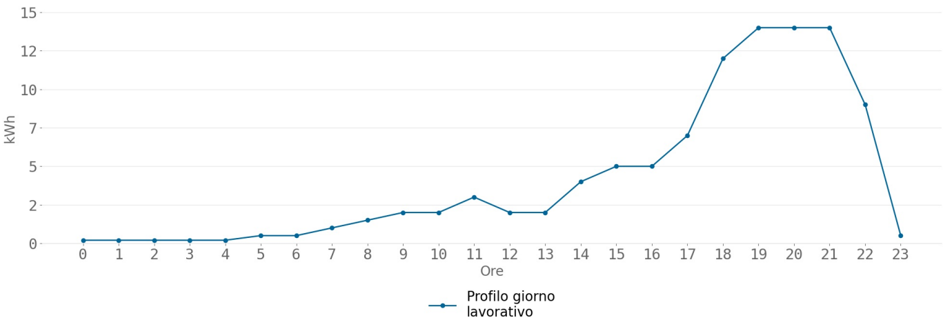
Profilo di consumo orario: CER_Fluminimaggiore (Campo_Sportivo)
